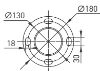
Рис. 3. Чертеж и габаритные размеры фланца OXOR-OK1-D100
