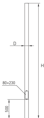
Рис. 1. Чертеж и габаритные размеры опоры OXOR-OT1/OK1-D108/D100
