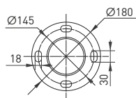
Рис. 2. Чертеж и габаритные размеры фланца OXOR-OT1/OK1-D108
