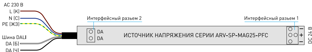
Рис. 1. Схема подключения
