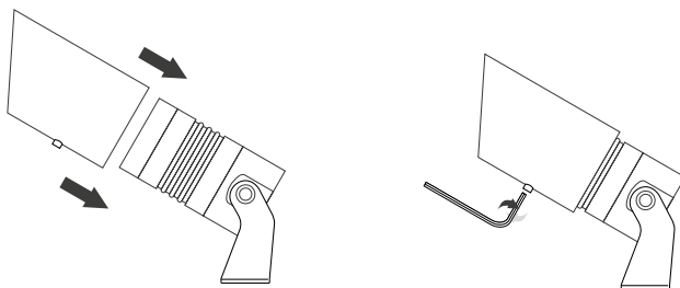
Рис. 1. Установка бленды на прожектор
